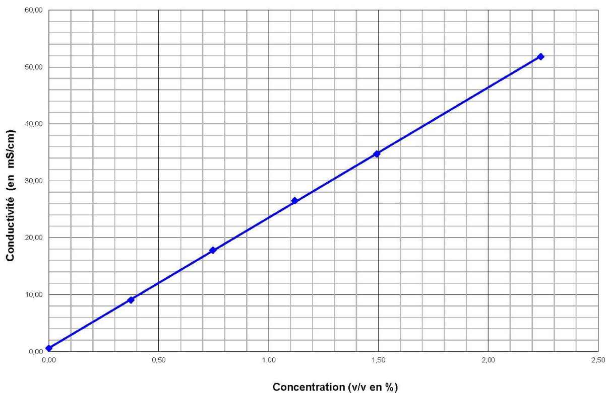
Courbe de conductivité à 25°C du CIP 3000 - V1 Courbe réalisée avec une eau de dureté = 11,7°f avec le conductimètre WTW Cond 3110
