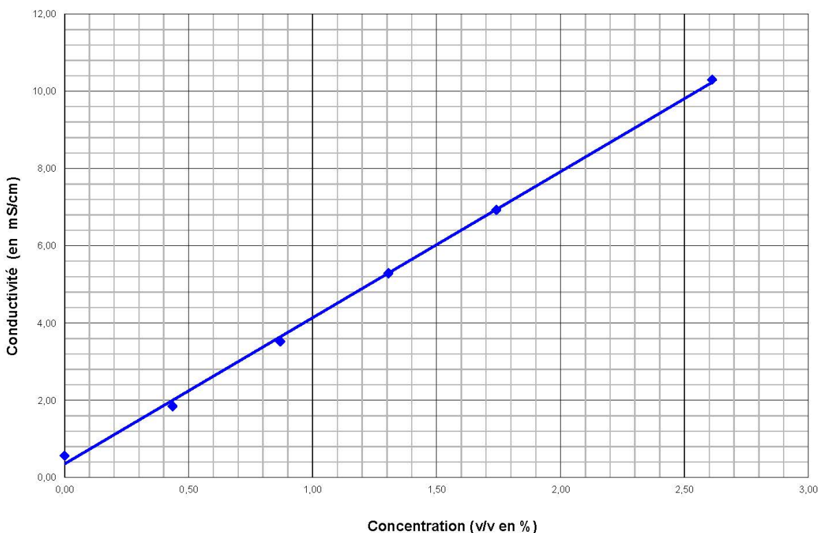
Courbe de conductivité à 25°C du CIP 1175 SI - V2 Courbe réalisée avec une eau de dureté = 21,9°f avec le conductimètre WTW Cond 3110
