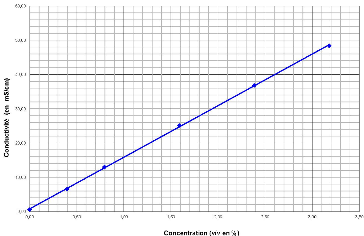
Courbe de conductivité à 25°C du CAM 1501 - V8 Courbe réalisée avec une eau de dureté = 17,7°f avec le conductimètre WTW Cond 3110
