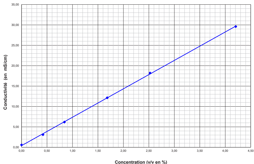
Courbe de conductivité à 25°C du DETERQUAT 4740 - V8 Courbe réalisée avec une eau de dureté = 22,8°f avec le conductimètre WTW Cond 3110
